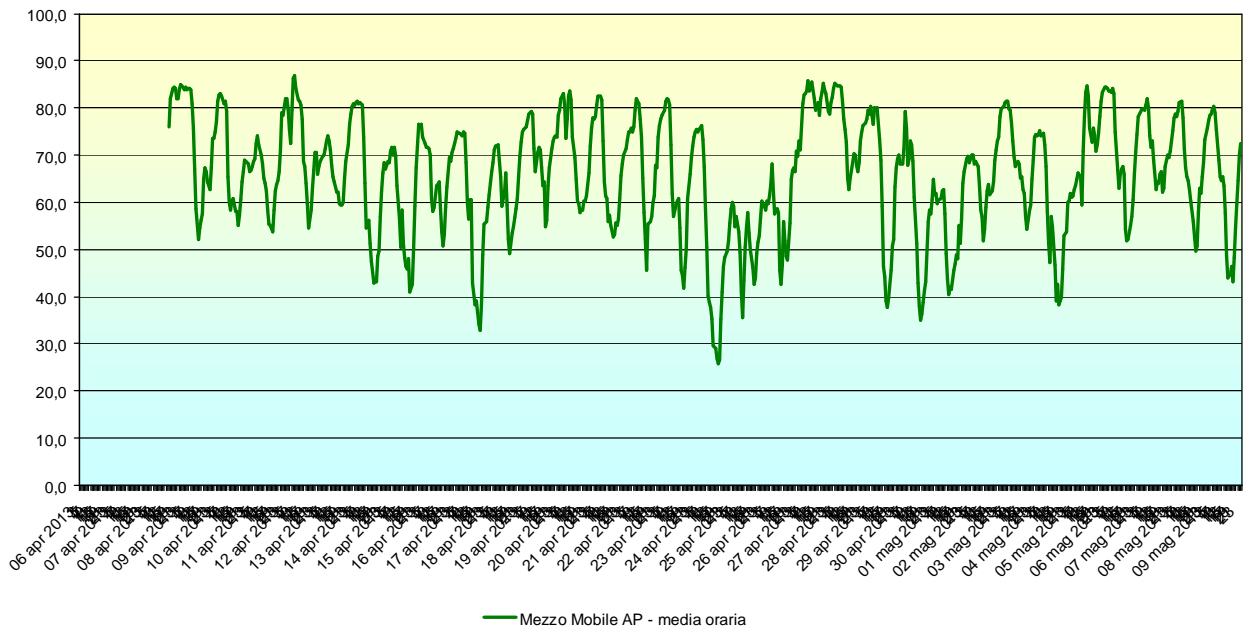
Parametro: U.R. (%), periodo: 06 apr 2013-09 mag 2013 - Dati validati
