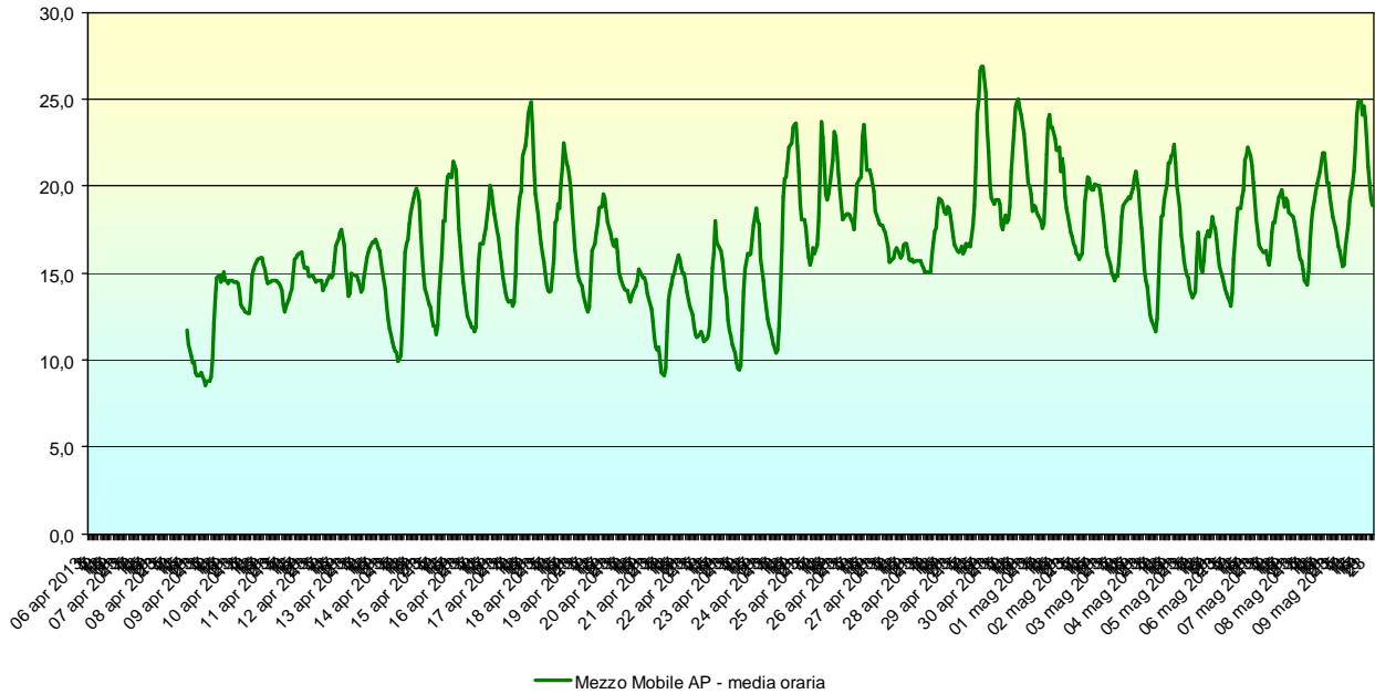
Parametro: Temp (°C), periodo: 06 apr 2013-09 mag 2013 - Dati validati
